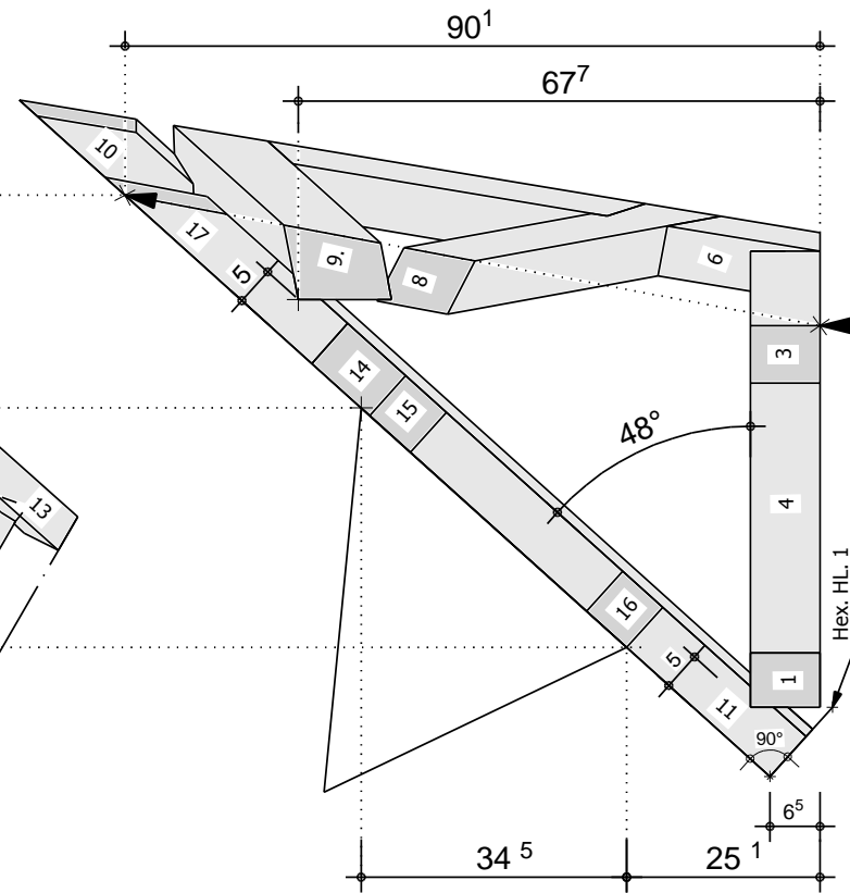
Schnitt A-A
